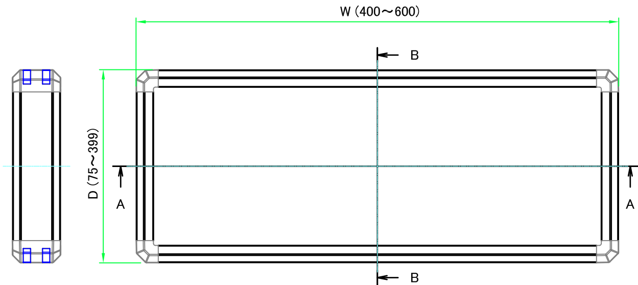
フレーム3側 / Frame3 side
