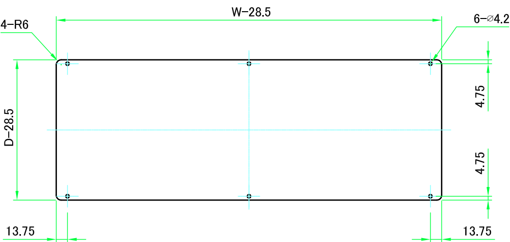
パネル裏面 / Panel Backside
