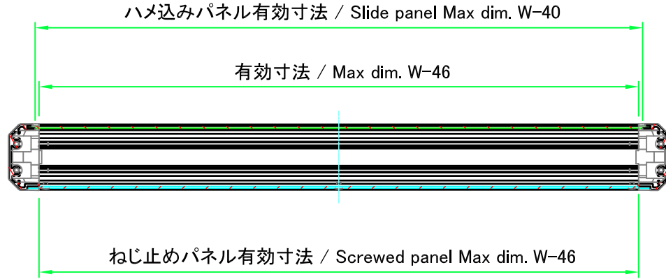
A-A ( 1 : 4 )
